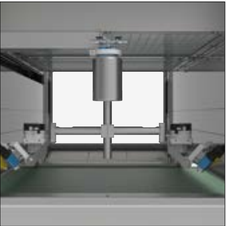
Braccio oscillante. Oscillating arm.
